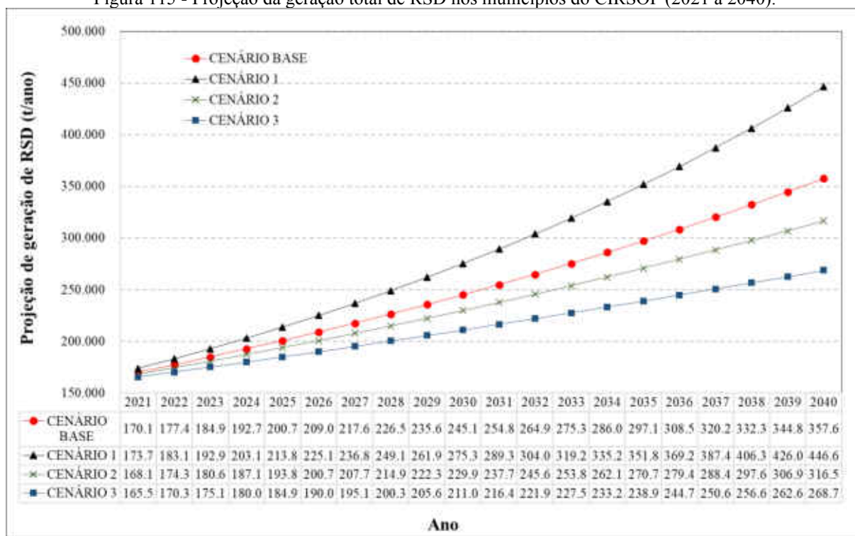
Figura 115 - Projeção da geração total de RSD nos municípios do CIRSOP (2021 a 2040).
