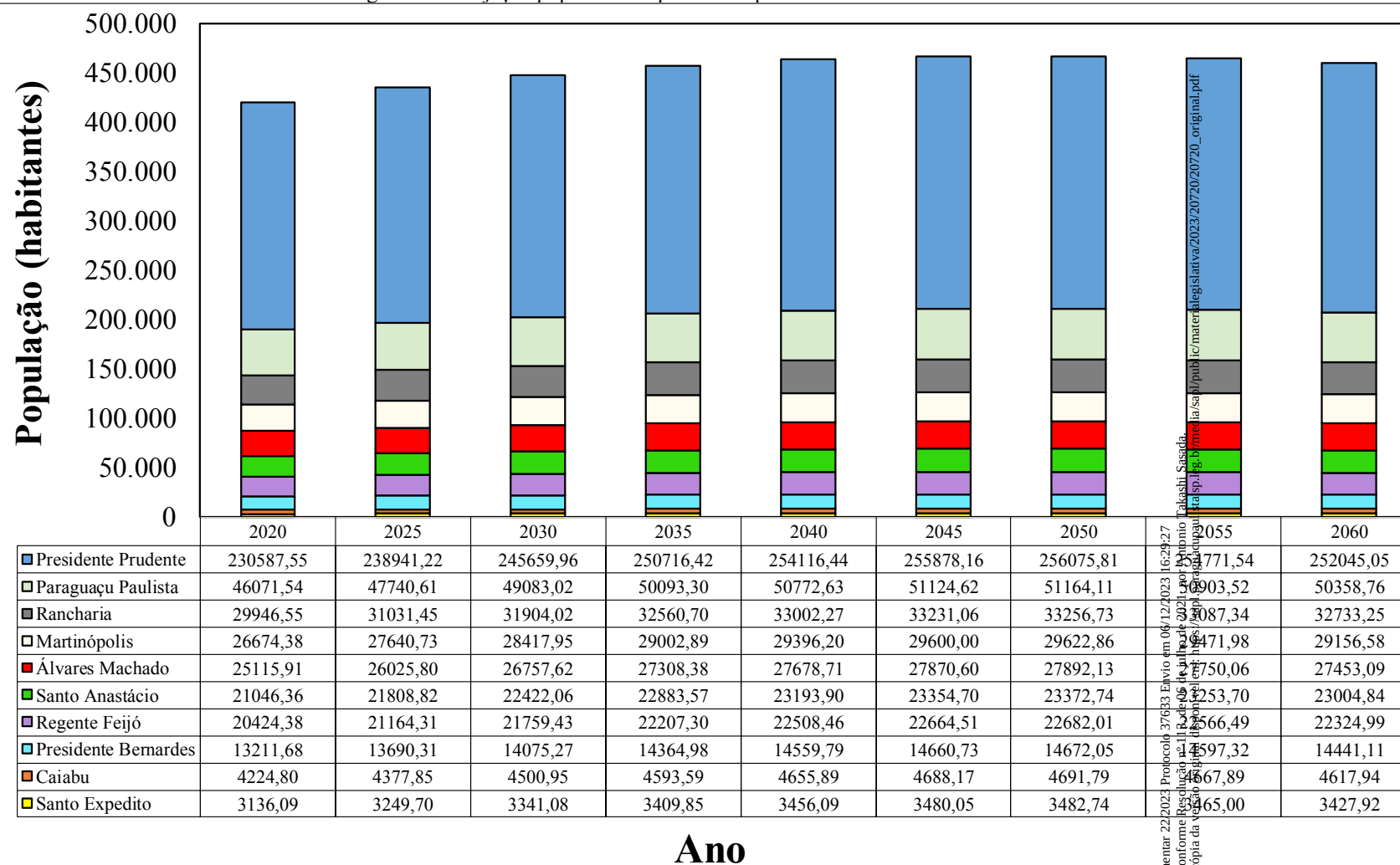
Figura 30 - Projeção populacional por município do CIRSOP até o ano de 2060.
