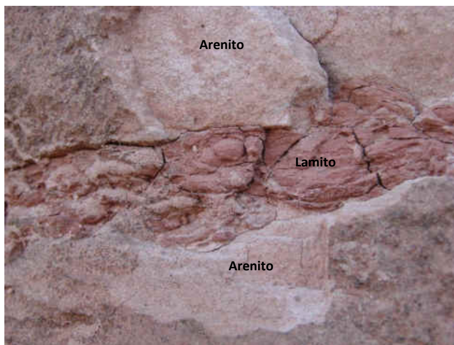
Figura 15 – Detalhe de afloramento do arenito com intercalação de lamito da Formação Presidente Prudente, na estrada Raimundo Maiolini na saída de Presidente Prudente em direção ao Distrito de Montalvão.
