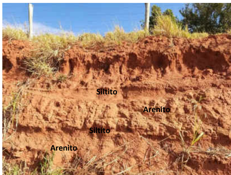
Figura 13 - Afloramento do arenito com intercalação de siltito da Formação Vale do Rio do Peixe, na estrada Raimundo Maiolini, entre os Distritos de Montalvão e Floresta do Sul.
