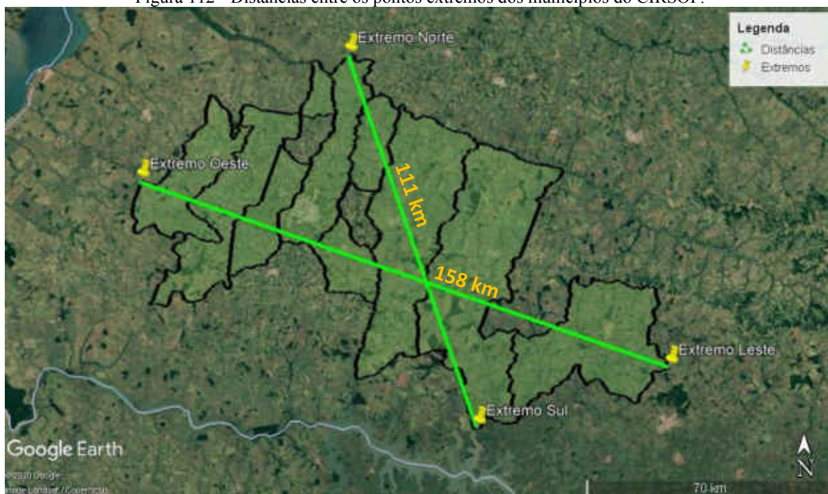
Figura 112 - Distâncias entre os pontos extremos dos municípios do CIRSOP.
