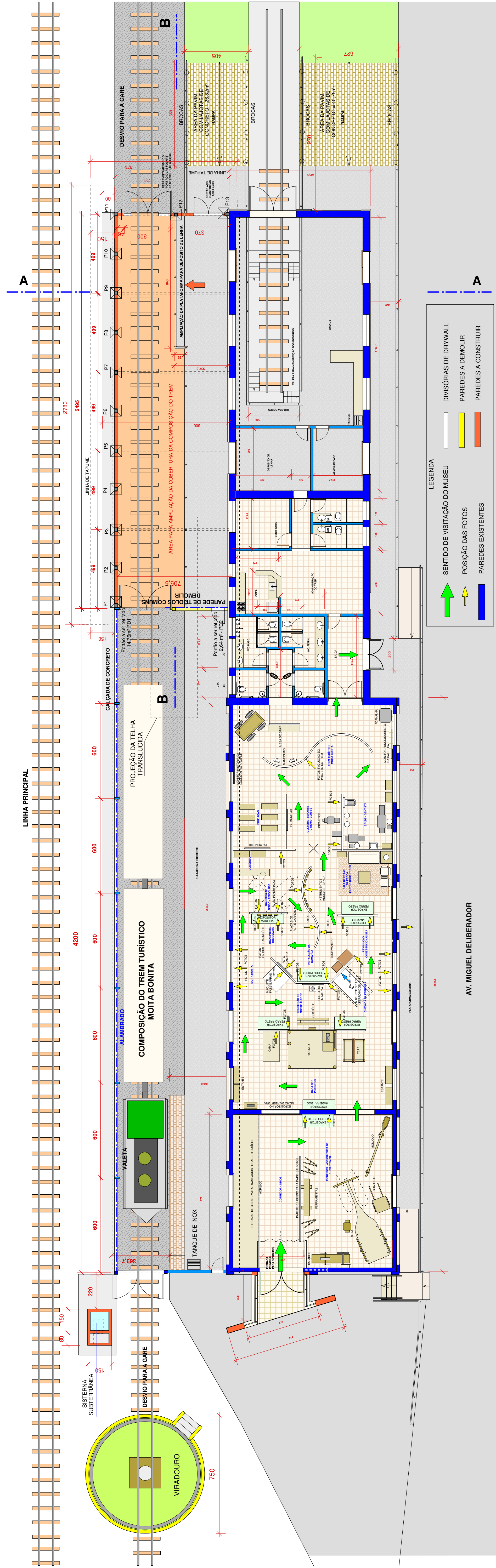
PROJETO PARA AMPLIAÇÃO DA GARE DO TREM TURÍSTICO - NP 420.616 ESC. 1:125
