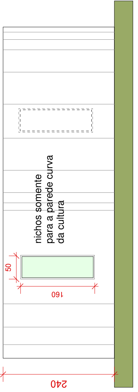
PAREDES PARA EXPOSITORES COM COMPENSADO DE MADEIRA SOBRE ESTRUTURA EM SARRAFO COM ACABAMENTO DE MASSA ACRÍLICA E TINTA LATEX ESC. 1: 50
